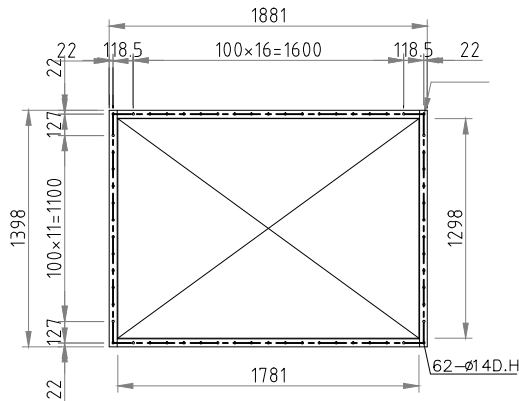
DISCHARGE COMPAISON FLANGE
