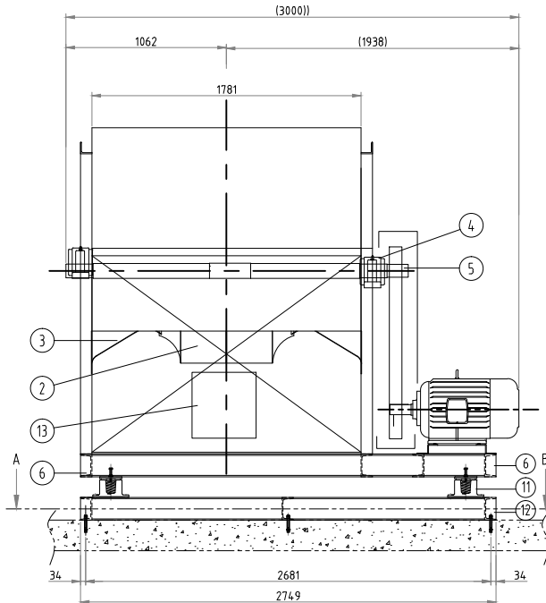
FAN FROUT VIEW
